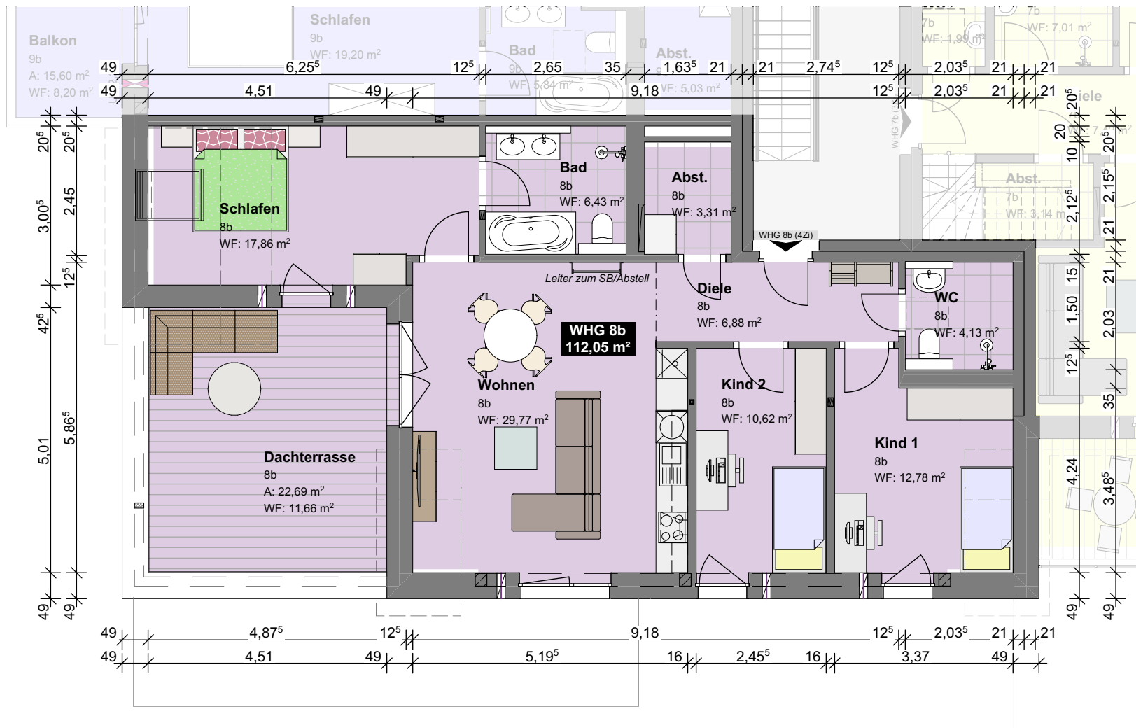
Dachgeschoss. Wohnung 8B
